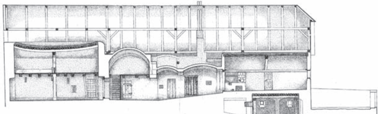
↗↑ Jaroslav Vajdiš: Vítějovice, rychta čp. 15, zaměření domu před jeho demolici: příčný a podélný řez, 1972.
